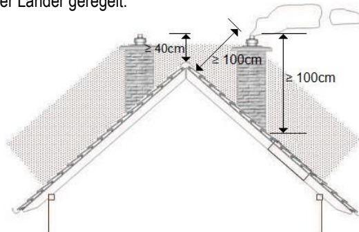
Abb. 2, Abgasanlagenhöhe über Dach, bei Dachneigungen ≥ 20 Grad
