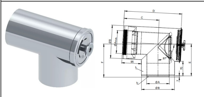
T-Anschluss 87° mit Revisionsdeckel und integriertem Kesselanschluss, Abgang „gleich“
