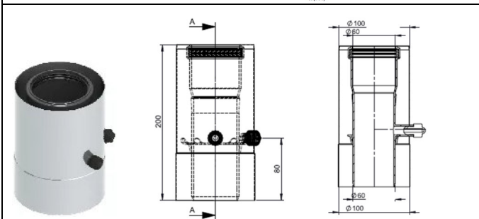
Messelement D60/100, Nutzlänge: 140 mm
