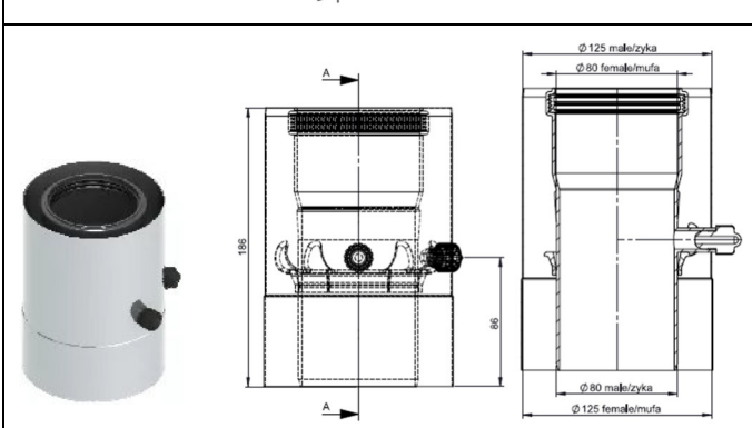
Messelement D80/125, Nutzlänge: 126 mm
