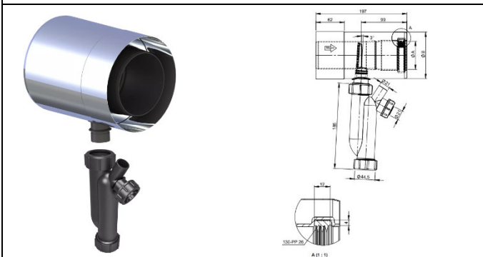
Kondensatablauf inkl. Siphon für horizontalen Einbau
