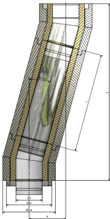
Variante Schachtlängen L=600 /1200mm
