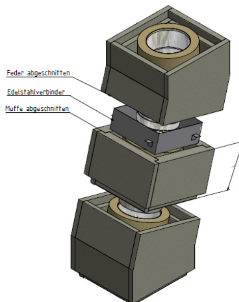
Variante Schachtlängen L=200/400/800/1000mm
