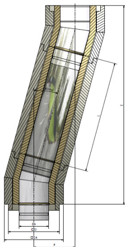
Variante Schachtlängen L=600 /1200mm
