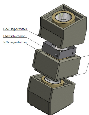
Variante Schachtlängen L=200/400/800/1000mm
