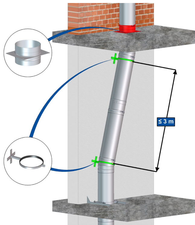
Bild 5-14: Schrägföhrung Wäscheschacht
