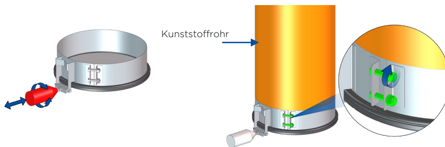
Bild 5-16: Selbstschließender Verschlussdeckel, zur nachträglichen Montage z. B. an Kunststoffrohr
