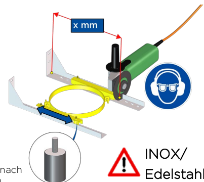
Bild 5-13: Konsole schallentkoppelt
