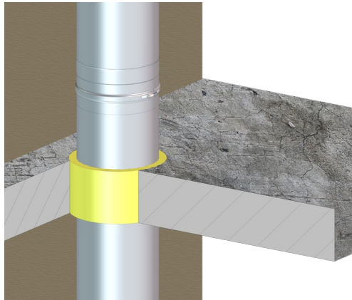
Bild 6-1: Dämmung Deckendurchbruch
