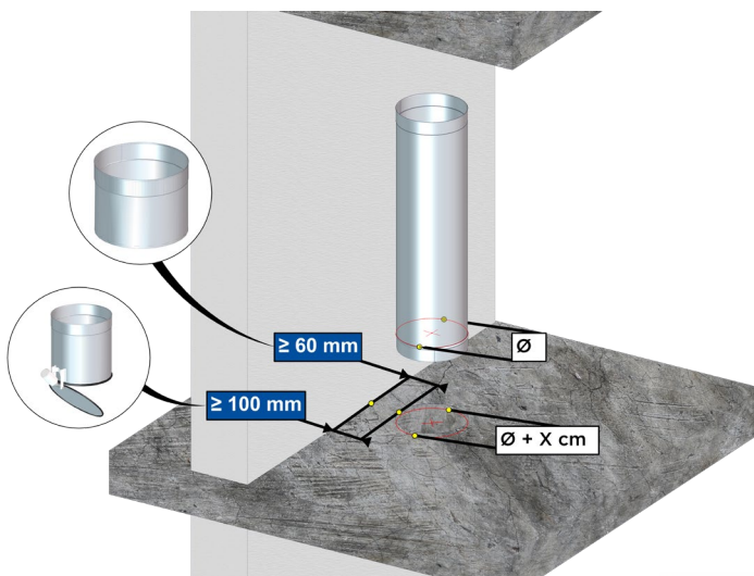
Bild 4-1: Größe Deckendurchbruch
