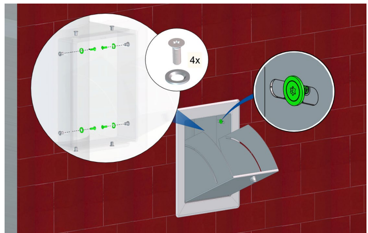
Bild 5-24: Befestigung Türen
