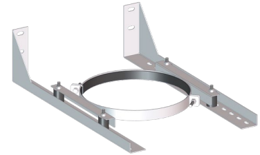
Bild 5-12: Konsole schallentkoppelt
