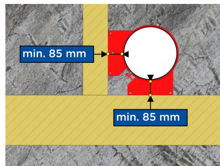
Bild 5-11: Wandabstände Konsolen im Rohbau
