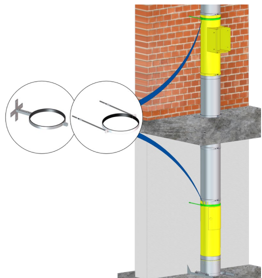
Bild 5-21: Befestigung Einwurfschächte mit Wandabstandshalter
