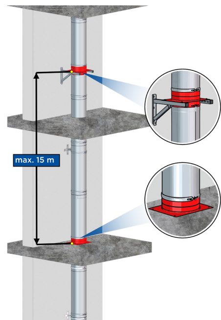
Bild 5-3: maximaler Abstand von Zwischenstützen
