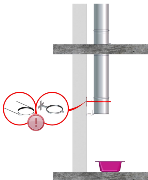
Bild 5-6: Wandabstandshalter am Auswurfelement anbringen
