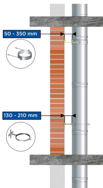
Bild 5-7: mögliche Wandabstände
